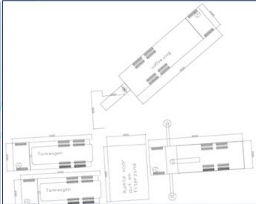
Voorbeeld booropstelling WKO-bron met bovengrondse afwerking [bron: GEBO (B)]
